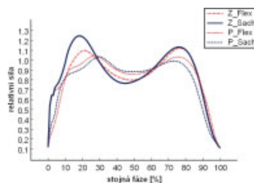
Graf 2. Grafické porovnání velikosti zatížení chodidla při chůzi na zdravé a protetické končetině.
